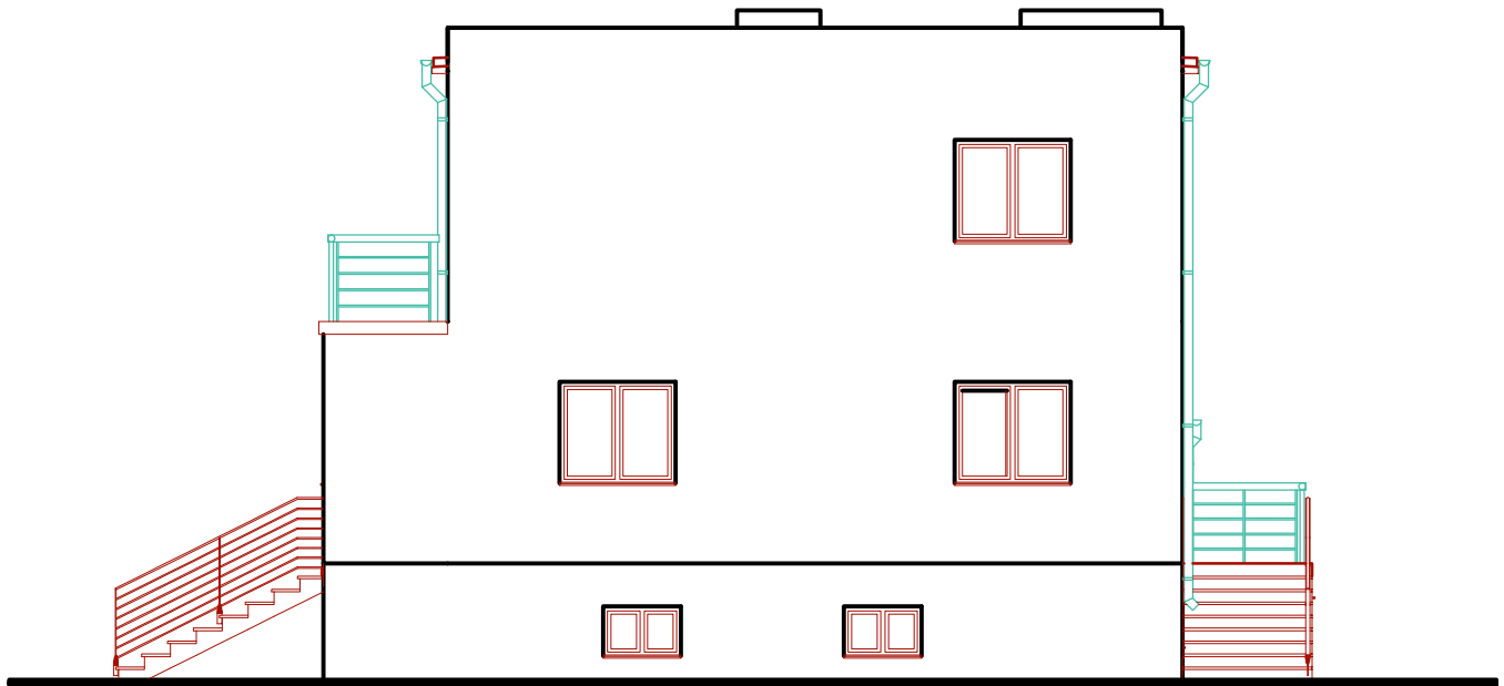
Elewacja południowa – inwentaryzacja
