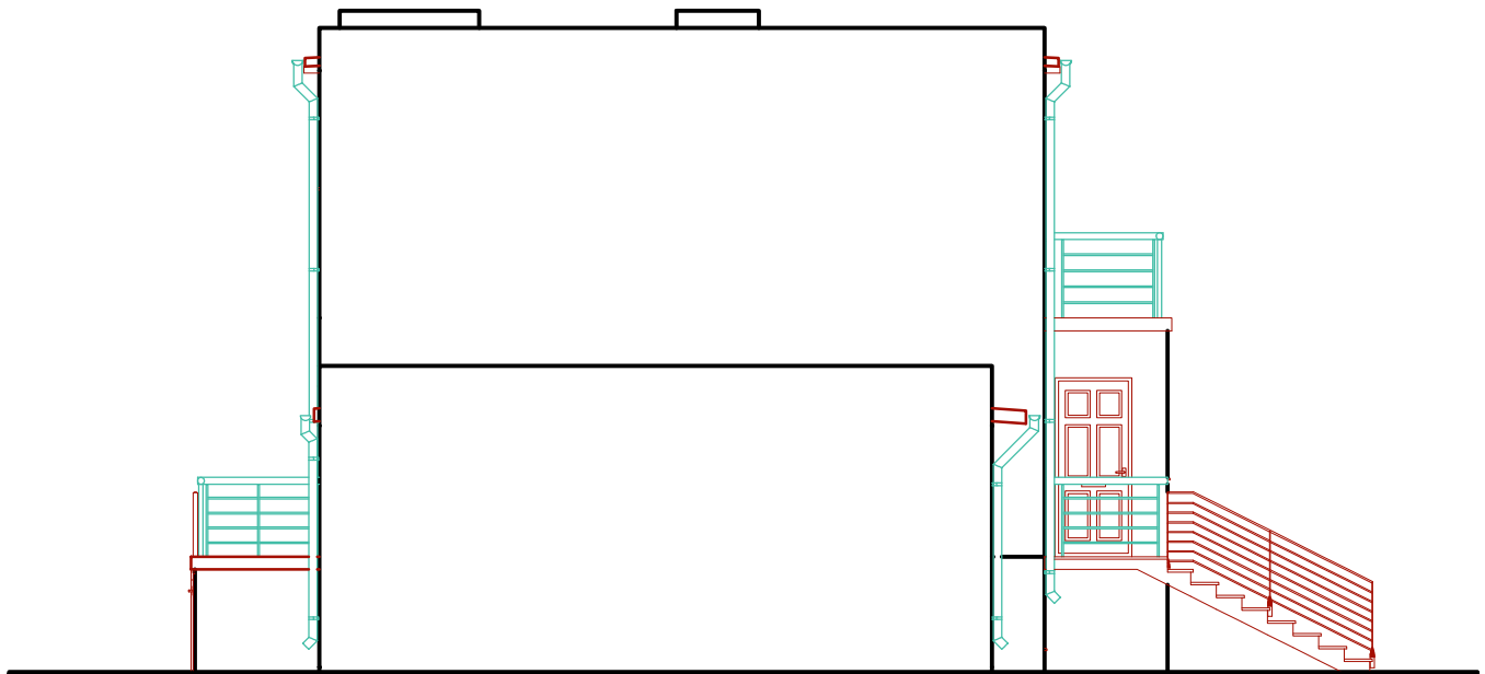
Elewacja północna – inwentaryzacja
